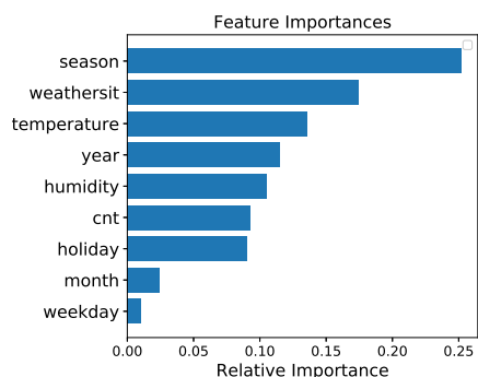
(d) Feature ranking from random forest model.
