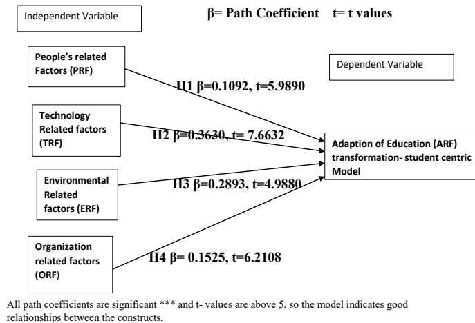
Fig.8. PLS-SEM Validation
