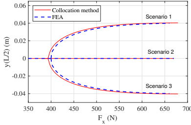
(b) F_x - y(L/2)
