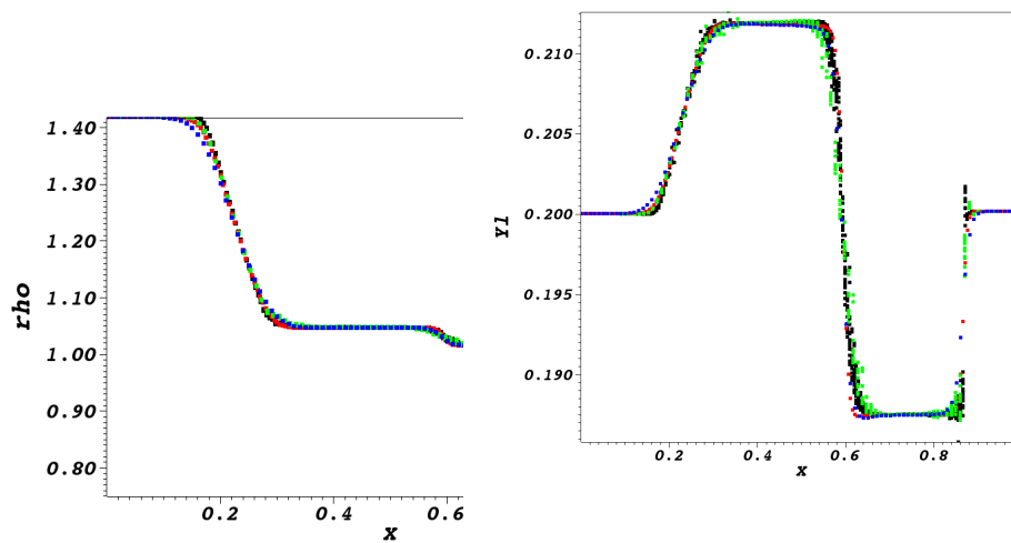
Fig. 13 Profil de la densité \rho (à gauche) et de la fraction massique de liquide Y_l (à droite) d'un tube à choc eau-vapeur en 2D (noir : 200x20 nœuds rd, rouge : 200x20 nœuds Clawpack, vert : 100x10 nœuds rd, bleu : 100x10 nœuds Clawpack)
