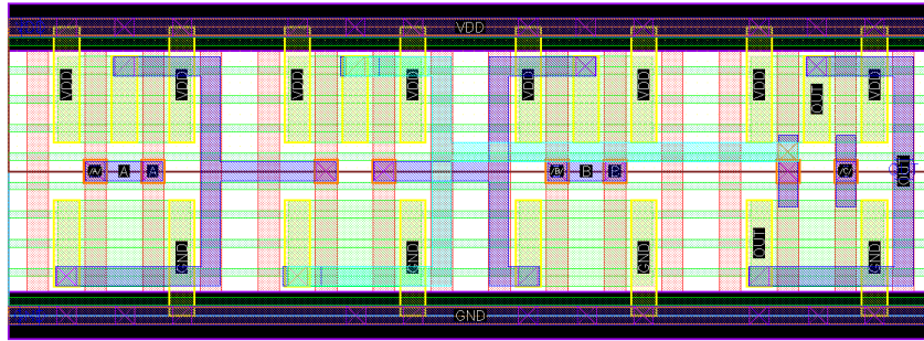
(b) OAI21_NAND
