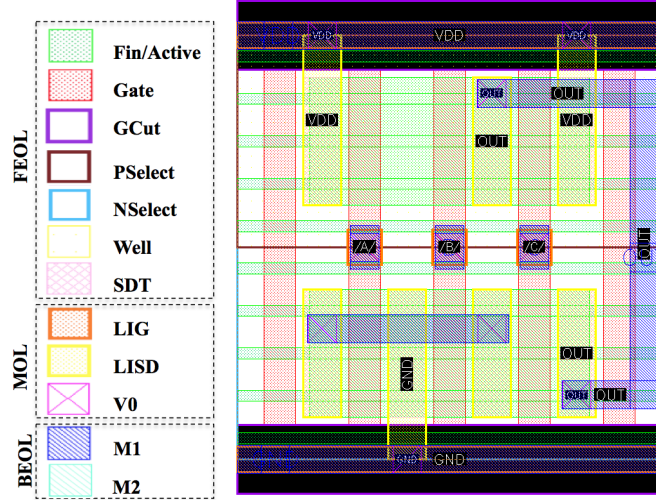
(a) OAI21
