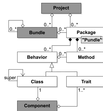
Fig. 15 The data meta-model
