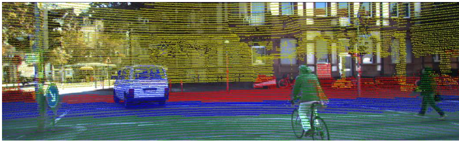
Fig. 4. RGB-D Data
