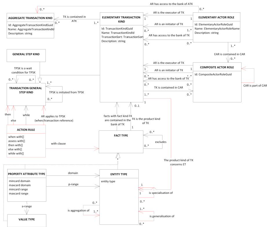
Fig. 5. DEMOSL data-meta-model
