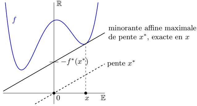
Fig. 3.6. Interprétation de f^*(x^*)
