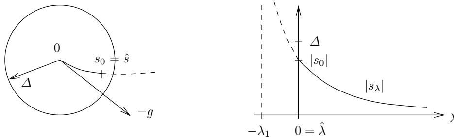
Fig. 9.3. Le cas A-1.
