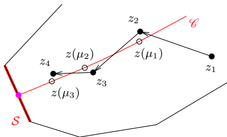
Fig. 18.1. Poursuite d'un objectif fuyant
