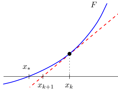
Fig. 10.1. Une itération de Newton
