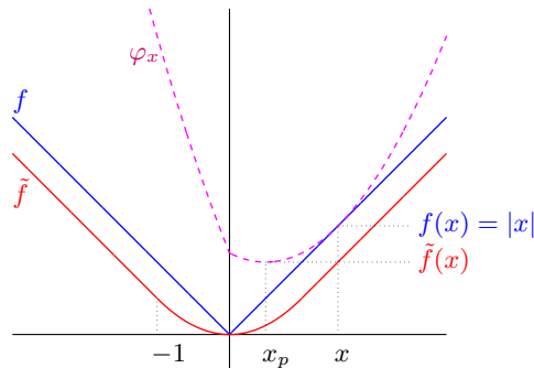
Fig. 3.10. Régularisée de Moreau-Yosida \tilde{f} de f : x \mapsto |x|
