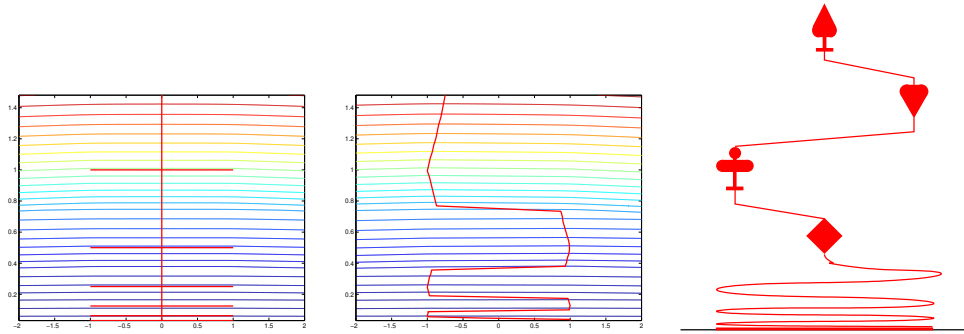
Fig. 16.4. Exemples de chemins centraux indésirables
