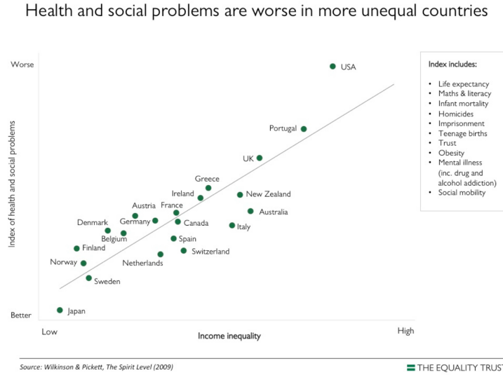
Fig. 19.1. Dépendance affine « la plus proche » de 21 couples (indice des problèmes sanitaires et sociaux, inégalités de revenus), avec un couple par pays considéré.
