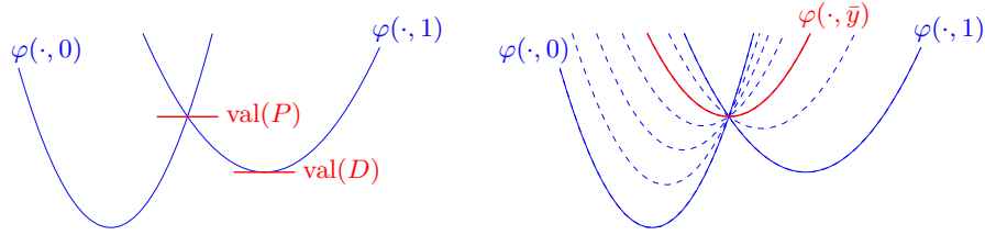
Fig. 14.1. Exemples avec et sans saut de dualité : \varphi(x, y) = 2(1 - y)[(x + 1)^2 - 1] + y[(x - 1)^2 - 1] . À gauche, Y = \{0, 1\} : il y a un saut de dualité car aucune des fonctions \varphi(\cdot, y) n'a pour valeur minimale \text{val}(P) . À droite, Y = [0, 1] : il n'y a pas de saut de dualité car pour \bar{y} = 2/3 , \varphi(\cdot, \bar{y}) a pour valeur minimale \text{val}(P) ; la solution duale est donc \bar{y} .
