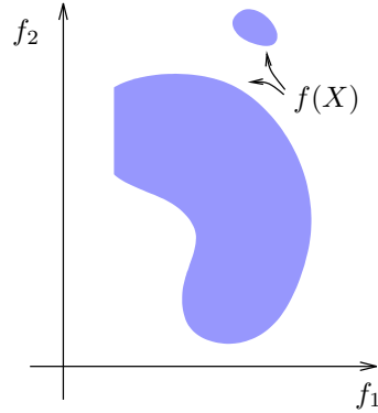
Fig. 3.13. Un ensemble f(X) dans \mathbb{R}^2
