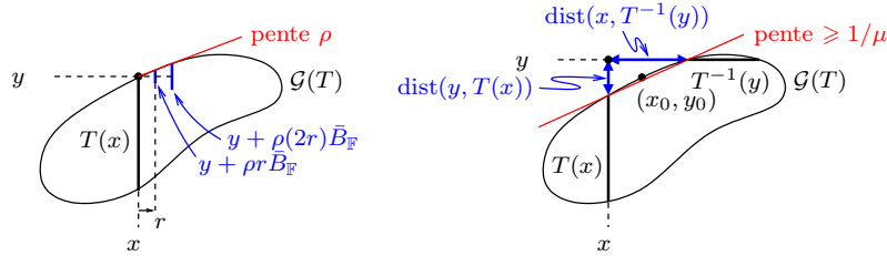
Fig. 4.6. Illustration des notions de multifonction ouverte de ratio \rho (à gauche) et de régularité métrique de module \mu (à droite) : les deux notions décrivent la variation de T(x) avec x , la première le fait de l'intérieur au graphe, la seconde le fait de l'extérieur ; ce ne sont pas des notions infinitésimales
