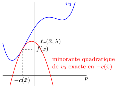
Fig. 14.3. Illustration de la proposition 14.33
