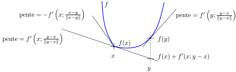
Fig. 3.4. Caractérisations de la convexité
