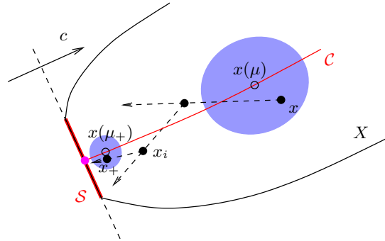
Fig. 16.3. Algorithme des grands déplacements
