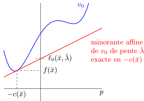
Fig. 14.2. Illustration de la proposition 14.27
