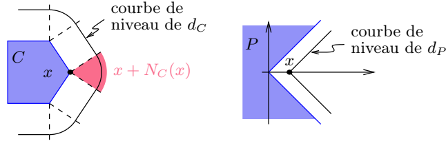
Fig. D.2. Différentiabilité de d_C et non-différentiabilité de d_P
