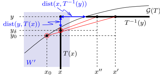
Fig. 4.7. Illustration de la démonstration de l'implication (iii) \Rightarrow (iv) du théorème 4.63
