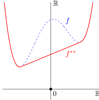
Fig. 3.7. Fonction biconjuguée f^{**} (en trait plein) de la fonction f de la figure 3.6 (en tirets)
