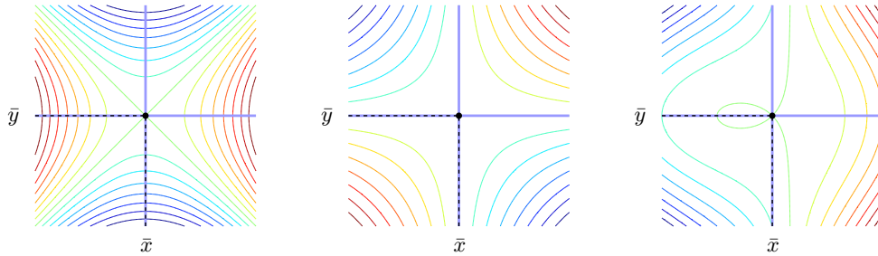
Fig. 3.11. Courbes de niveau de fonctions \varphi avec point-selle (\bar{x}, \bar{y}) = (0, 0) : \varphi(x, y) = x^2 - y^2 à gauche, \varphi(x, y) = xy au milieu et \varphi(x, y) = (x + y)(x - y) + (x + y)^3 + (x - y)^3 à droite.
