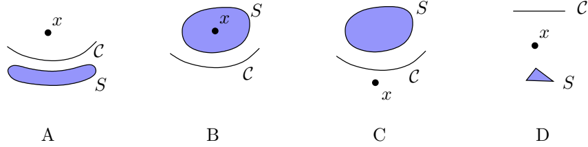
Fig. 3.14. Représentation du sous-différentiel d'une fonction convexe ?
