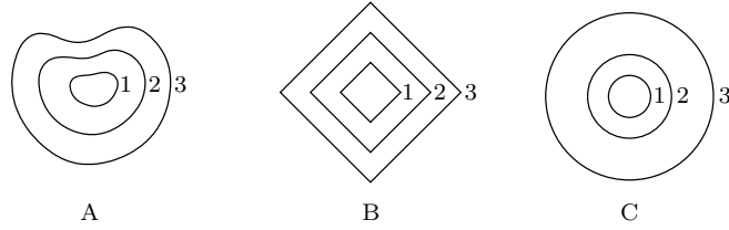
Fig. 3.12. Courbes de niveau d'une fonction convexe ?
