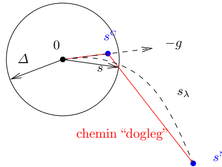
Fig. 9.8. L’algorithme « dogleg » de Powell (on a translaté x en 0).
