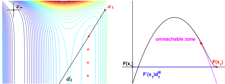
Fig. 10.3. Itérés de Newton avec recherche linéaire pour le système (10.16)
