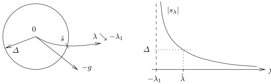
Fig. 9.5. Le cas B-1.
