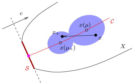
Fig. 16.2. Algorithme des petits déplacements
