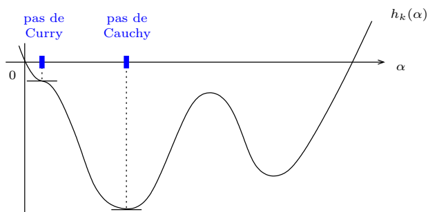
Fig. 6.2. Règles de Cauchy et de Curry.
