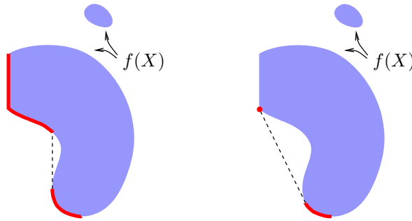
Fig. D.1. Image par f des points Pareto optimaux (g) et moyennement optimaux (d)
