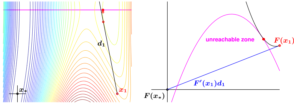
Fig. 10.2. Itérés de Newton avec recherche linéaire pour le système (10.15)
