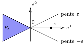
Fig. D.3. Illustration d'une constante de Hoffman tendant vers +\infty (exercice 17.14)
