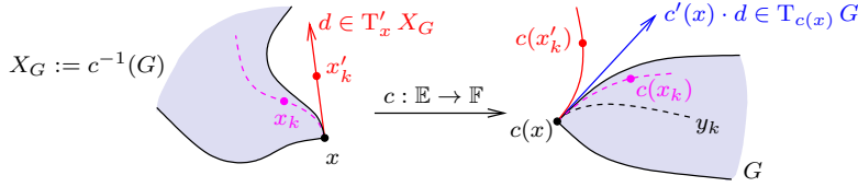
Fig. 4.8. Illustration de la démonstration de (4.71a) pour établir la proposition 4.69
