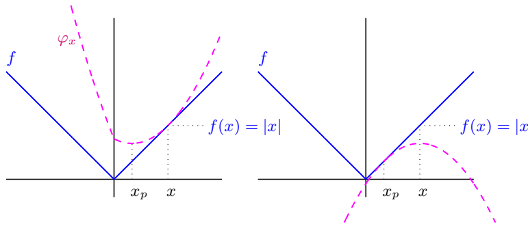
Fig. 3.9. Deux points de vue sur le point proximal associé à la fonction f = |\cdot|
