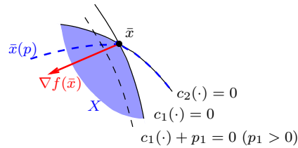
Fig. 4.9. Interprétation marginaliste des multiplicateurs optimaux
