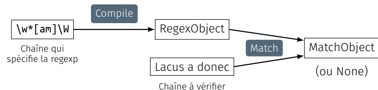
FIGURE 9.2 — Workflow d'une expression régulière.
