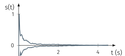
FIGURE 4.7 — Forme d'onde et spectre d'une note C 4 de violon jouée pizzicato (5 ms).
