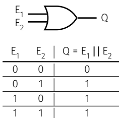
FIGURE 4.2 — Représentation et table de vérité de porte logique « OU » (notation étasunienne la plus usitée; voir comparatif avec la notation européenne).
