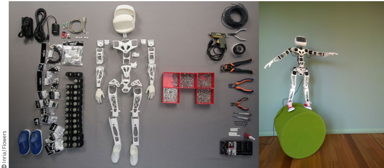
FIGURE 3.4 — POPPY a été développé à l'INRIA. Ce robot, en open source (tous ses composants sont publics), aide à explorer les mécanismes du développement cognitif des enfants. Il est aussi utilisé pour l'éducation des écoliers et des collégiens.
