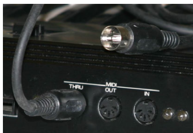
Triplet classique des ports MIDI IN, OUT et THRU en connectique DIN.
