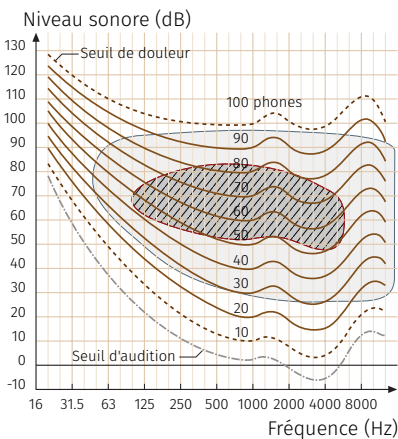
FIGURE 4.18 — Courbes d'isophonie binaurale (en phons) et champs audibles de la parole (—) et de la musique (---).
