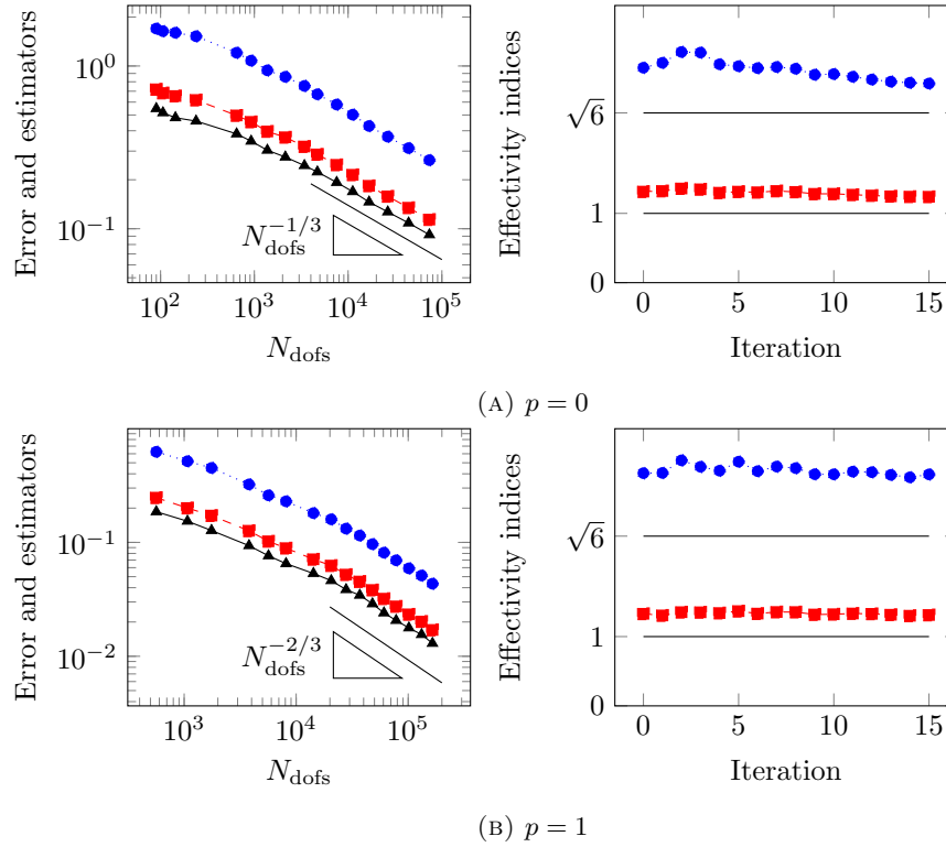
FIGURE 6.7. Fichera domain example
