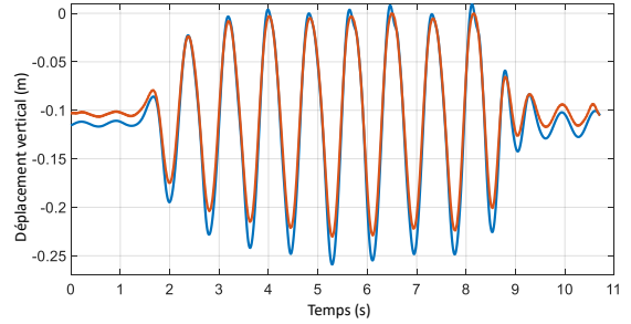
Figure 2: Déplacements verticaux expérimental (bleu) et numérique (rouge) en x = L
