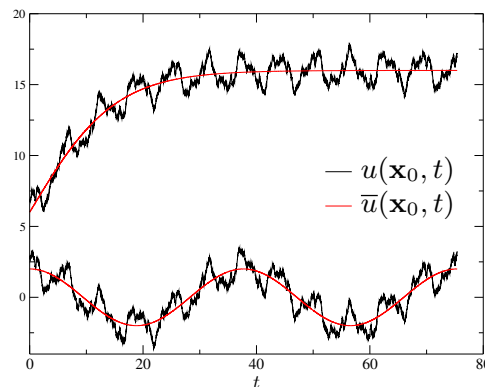
Exemples de signaux mesurés en écoulements turbulents transitoires ou cycliques
