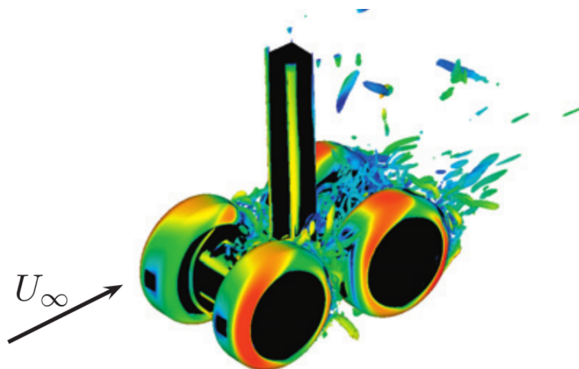
Simulation PANS de l'écoulement autour d'un train d'atterrissage rudimentaire (Iso-surfaces du critère Q colorés par l'amplitude de la vitesse)
