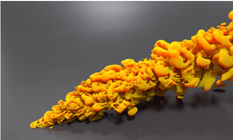
Jet en écoulement transverse (Iso-surfaces du critère Q)
