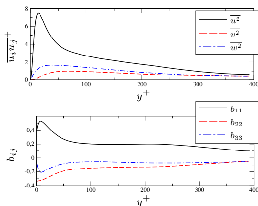
Données DNS de Kim et al. (1999) en canal à Re_\tau = 395
