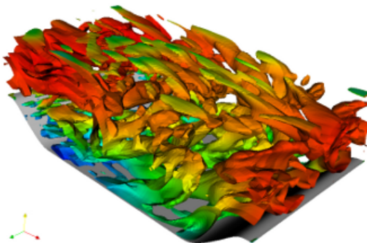
Écoulement au-dessus d'une colline périodique (Iso-surfaces du critère Q colorés par l'amplitude de la vitesse) Bentaleb & Manceau (2011).
