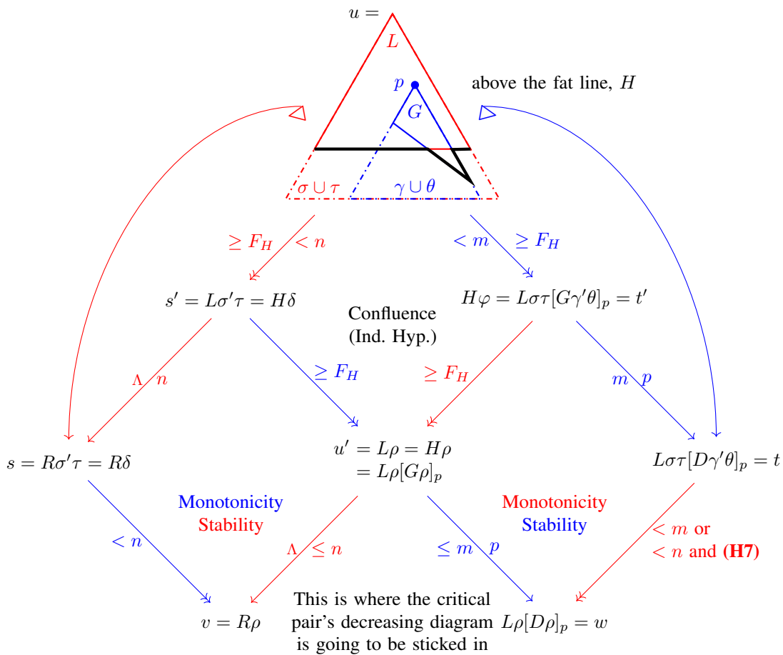
Fig. 2. Critical pair lemma: Lemma 10
