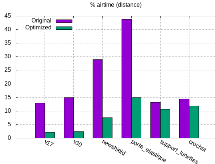
FIGURE 1 – Comparaison de la version non-optimisée et optimisée du pourcentage des déplacements à vide par rapport à l’ensemble des déplacements pour les différents modèles
