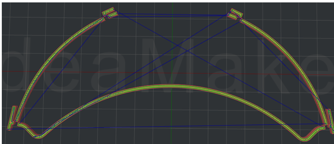
FIGURE 4 – Visière V30 - IdeaMaker 3.5.3.4250 - Déplacements à vide en bleu
