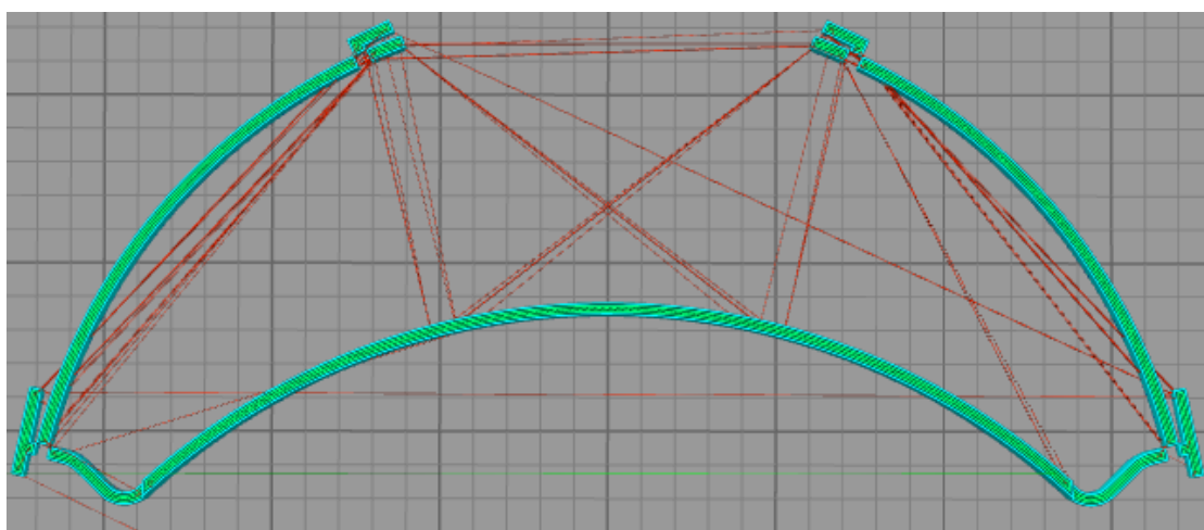
FIGURE 5 – Visière V30 - Simplify3D 4.1.2 - Déplacements à vide en rouge
