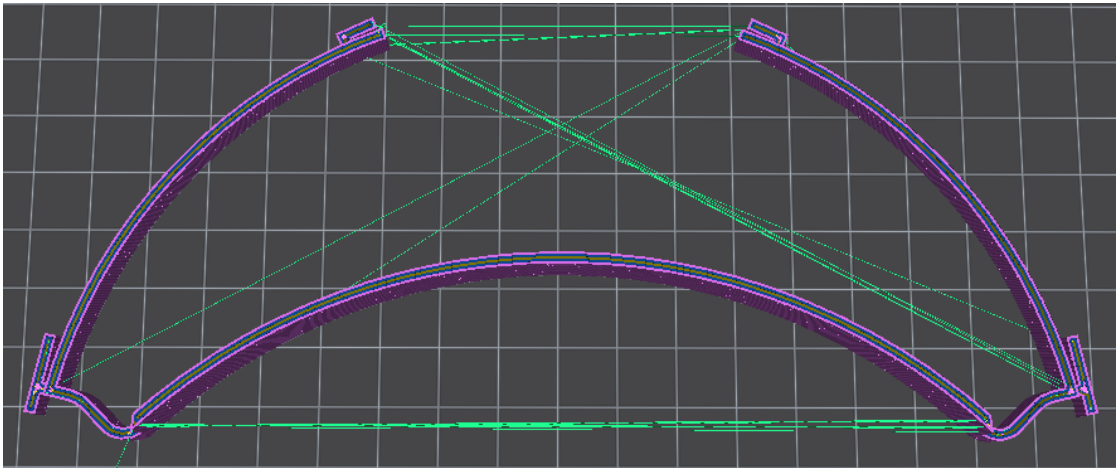
FIGURE 3 – Visière V30 - IceSL 2.3.4 - Déplacements à vide en vert
