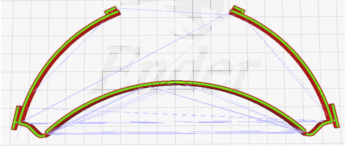
FIGURE 2 – Visière V30 - Ultimaker Cura 4.4.1 - Déplacements à vide en bleu
