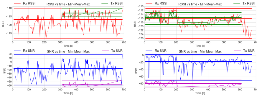
(a) RSSI & SNR ( SF=9 BW=125 kHz). (b) RSSI & SNR ( SF=12 BW=250 kHz).
