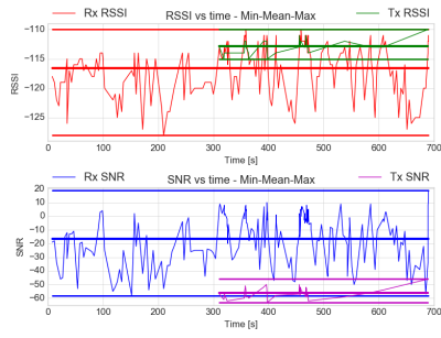
(e) RSSI &amp; SNR (SF=9 BW=125)
