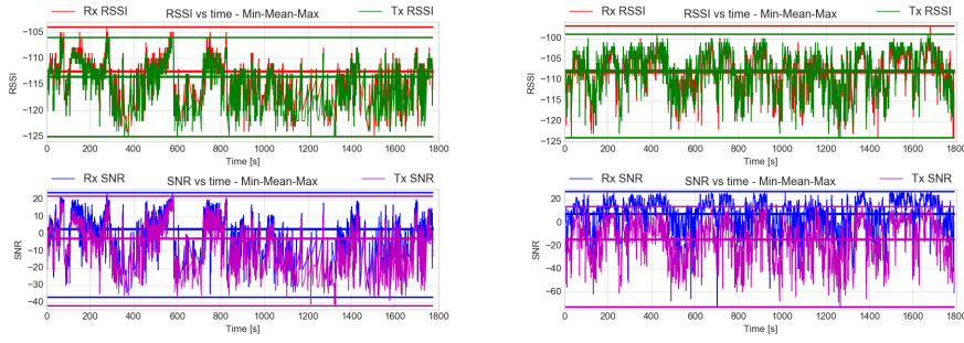
(a) RSSI & SNR (SF=7 BW=125 kHz). (b) RSSI & SNR (SF=11 BW=250 kHz).
