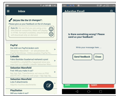
Fig. 3. Feedback prompts
