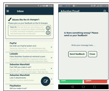
Fig. 3. Feedback prompts
