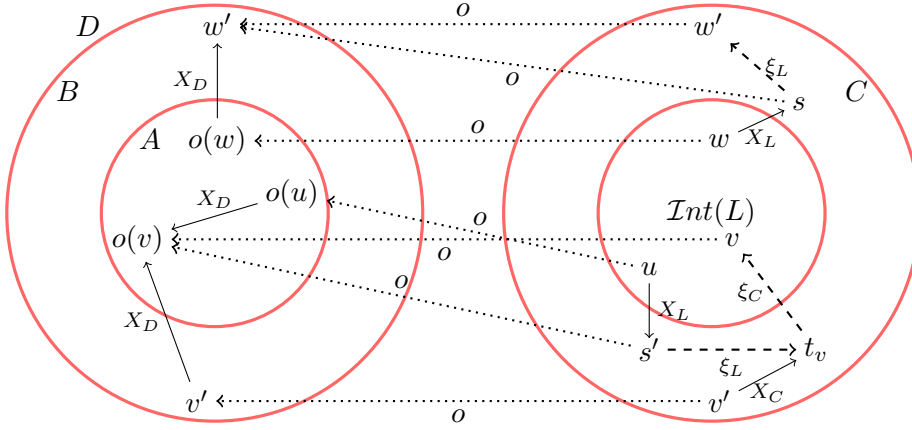
Fig. 3 Proof of Lemma 4
