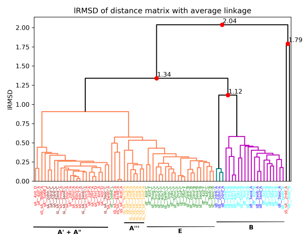
(D) Loop2 IRMSD
