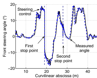
Fig. 15. Steering control
