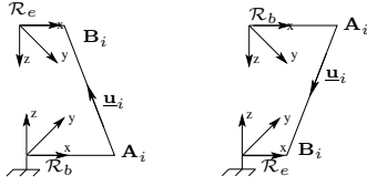
FIG. 2 – Dualité entre les deux modes : effecteur mobile et effecteur fixe.
