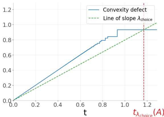
(d) Choice of t - Swissroll
