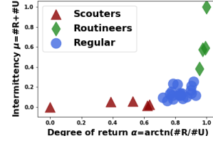
Figure 3: Privamov
