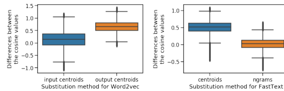
FIG. 2 – Différence entre la similarité cosinus obtenue avec les vecteurs originaux et ceux obtenus avec les substituts, pour Word2vec (gauche) et FastText (droite).
