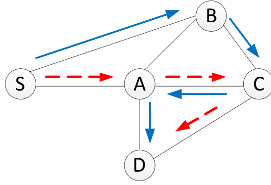
Fig. 3: Example of lemma 1
