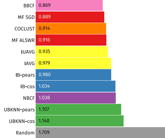
(b) ML-1M
