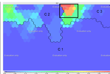
Fig. 5. SOM (eigenvector centrality)
