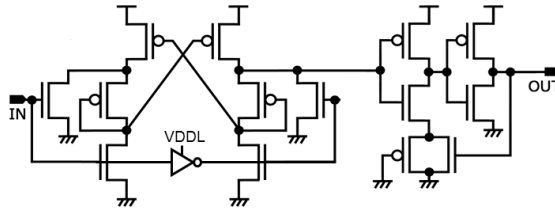
Fig. 5. LS circuit [16].
