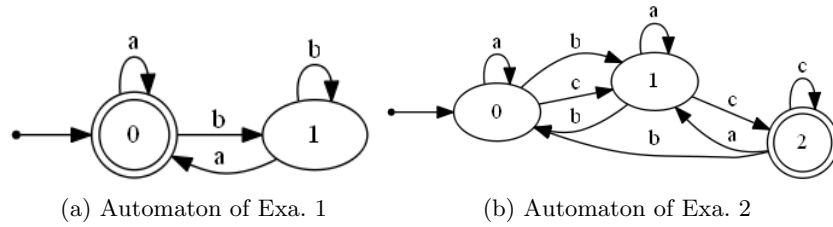
Fig. 5. Automata examples
