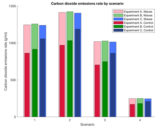
(d) Carbon dioxide emissions rate.
