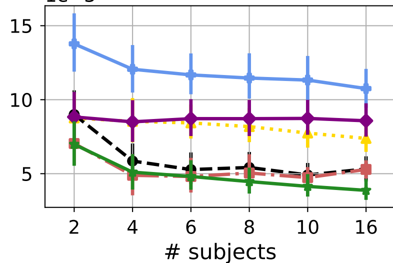
1e-3 MSE
