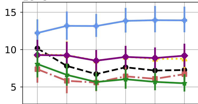
1e-3 MSE
