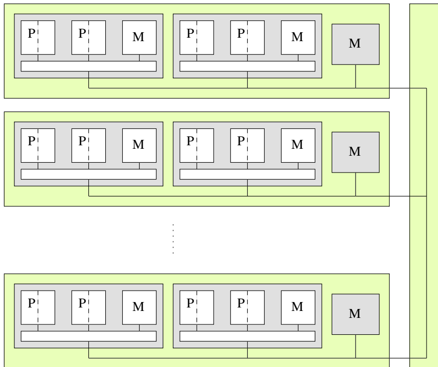
(a) Deux processeurs hyperthreadés et un peu de mémoire sur une même puce avec un niveau de cache, cette puce est implantée en deux exemplaires sur une même carte fille avec un peu de mémoire, et l'on enfiche enfin de telles cartes sur une carte mère.
