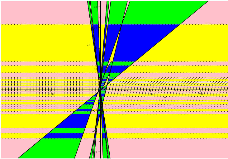
Fig. 4 Global view - Parameter space decomposition
