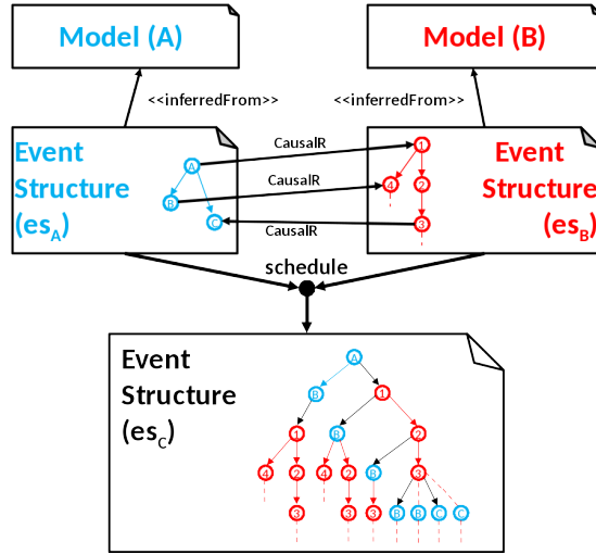
Fig. 6 \text{schedule}(es_A, es_B, \text{CausalR}) \Rightarrow es_C
