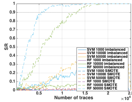
(d) Success rate (SR) on AES_RD dataset.
