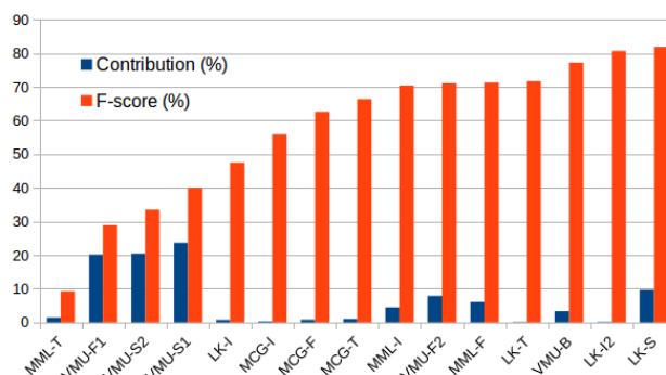
Figure 8. Contributions de chacun des systèmes dans la fusion mesurée par indice de Gini sur les forêt aléatoires, mis en regard de la F-mesure de ces systèmes ; évaluation par groupe de messages partageant un même contenu multimédia
