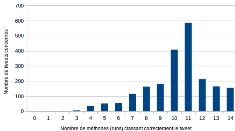
Figure 6. Histogramme des messages selon le nombre de méthodes les classant correctement; évaluation par groupe de messages partageant un même contenu multimedia
