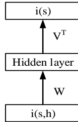
Fig.4. DAE
