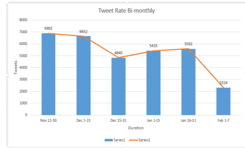
Fig. 2. Tweet rate for GST
