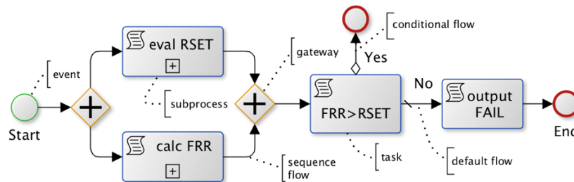
Fig. 2. Exemplar BPMN-compliant CDP
