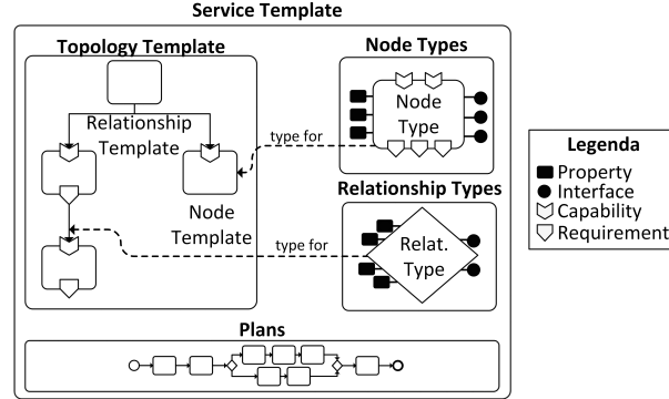
Fig. 1. TOSCA ServiceTemplate.
