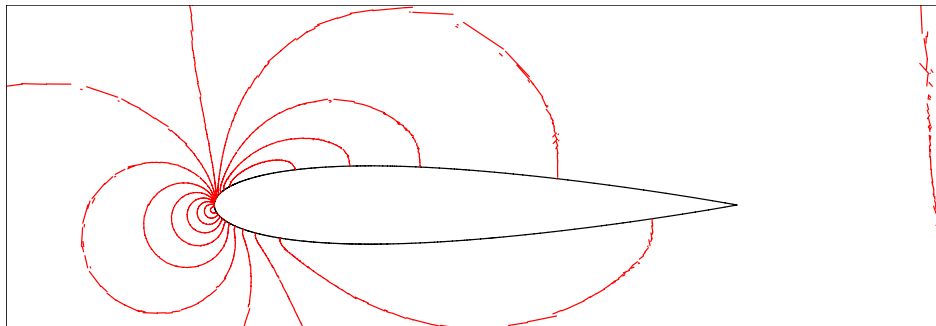
(b) NACA 0015
