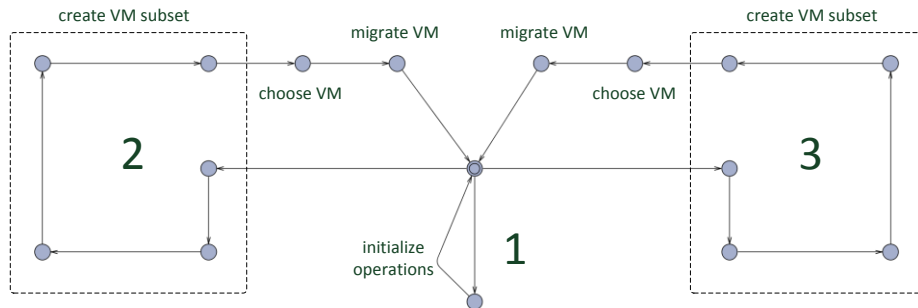
Fig. 5. PM automaton
