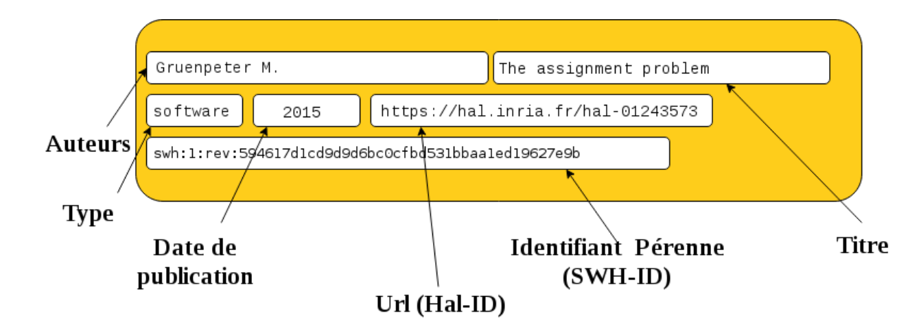
Figure 7: Le format de citation d'un logiciel[3]
