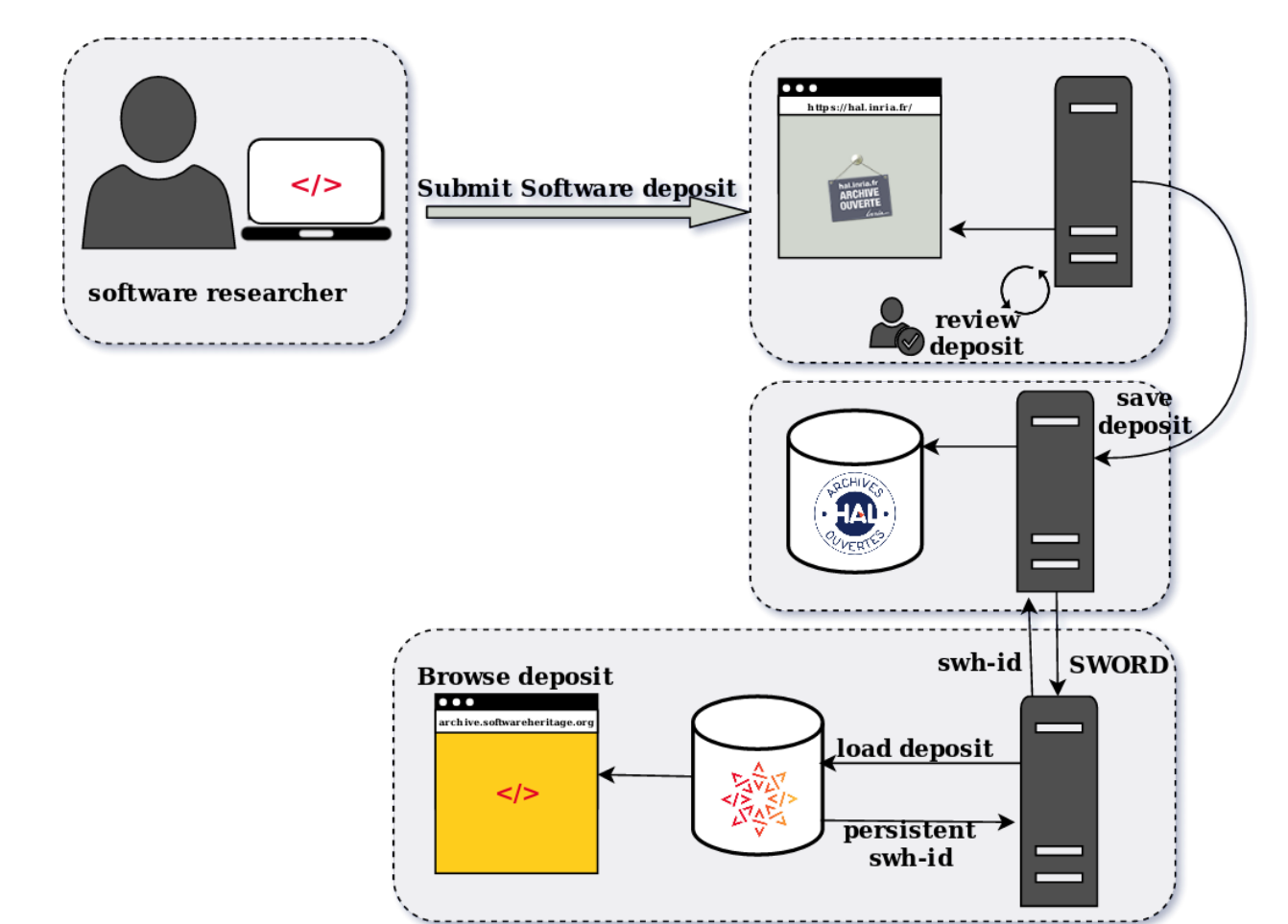
Figure 5: Le processus de dépôt et d'archivage
