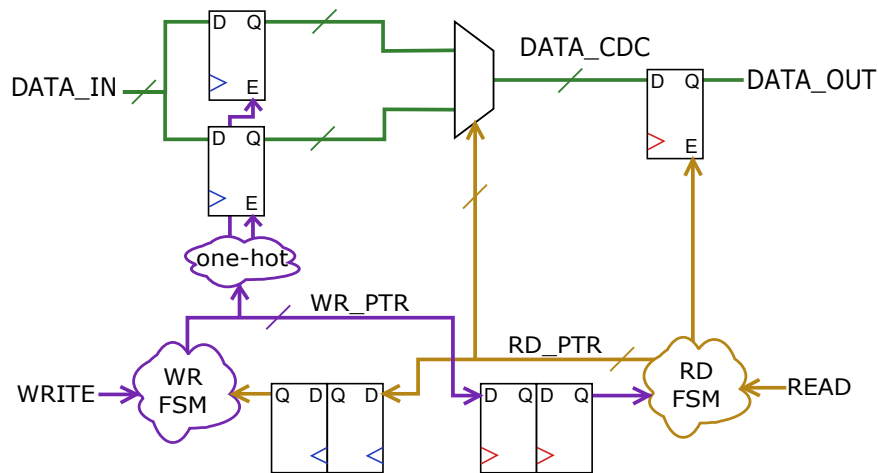
Fig. 7. FIFO synchronization
