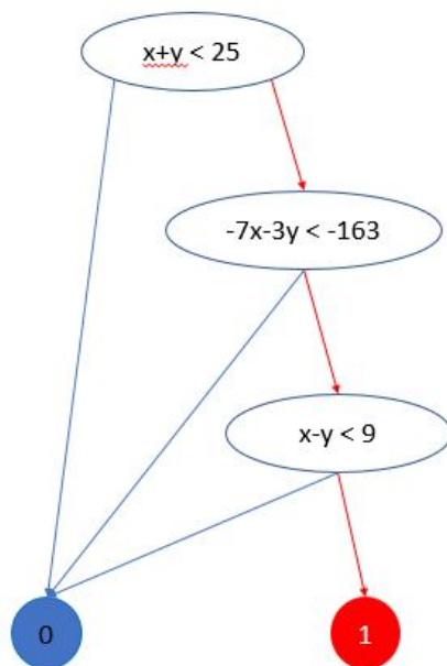
FIGURE 3.2: Représentation de F1 sous forme de LDDs + avec n = 3
