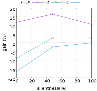
(b) bfs
