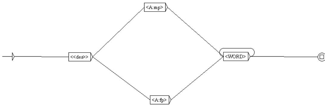
Figure 23 automate qui permet d'identifier le syntagme recherché : "des" + ADJ
