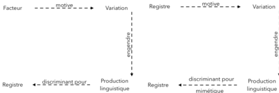
Figure 38 schéma de la motivation de la variation
