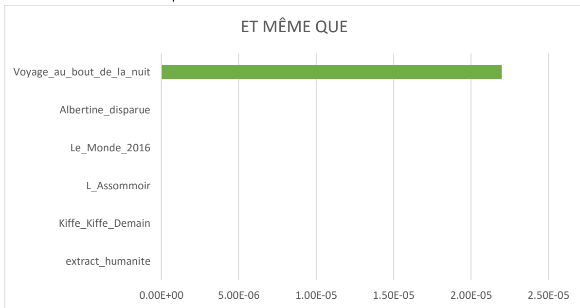
Figure 33 graphe des fréquences relatives du motif
