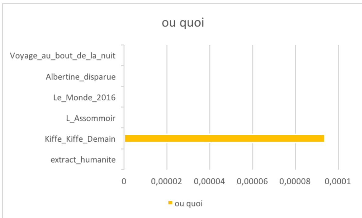
Figure 32 graphe des fréquences relatives du motif
