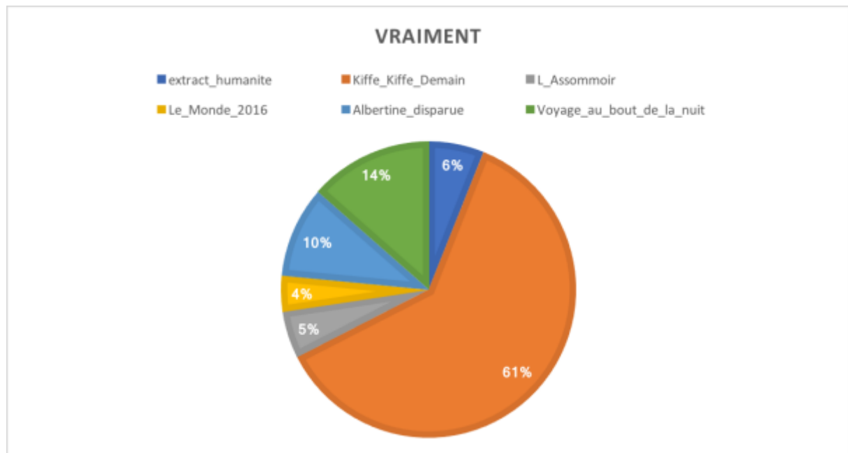
Figure 28 comparaison entre les textes/registres de la présence de "vraiment" dans ces derniers
