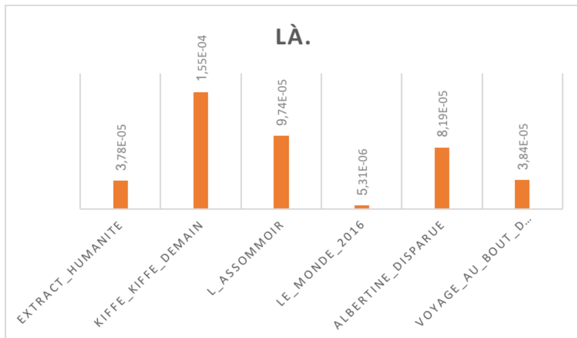
Figure 7 graphique des fréquences relatives des "là." c'est à dire en fin de phrase dans chaque œuvre/registre
