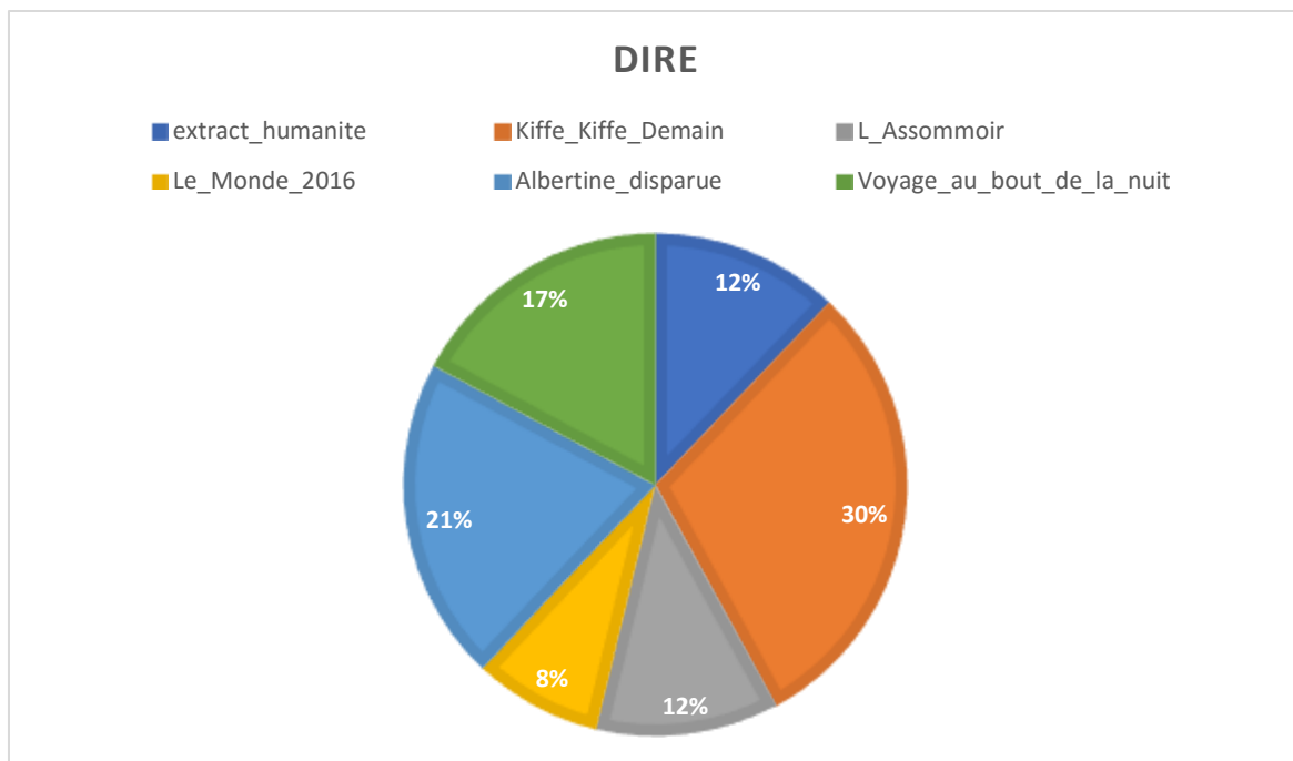
Figure 42 comparaison des fréquences relatives du lemme "dire" dans chaque registre
